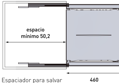
Espaciador para salvar bisagras incorporado
