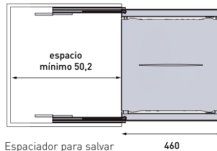
Espaciador para salvar bisagras incorporado
