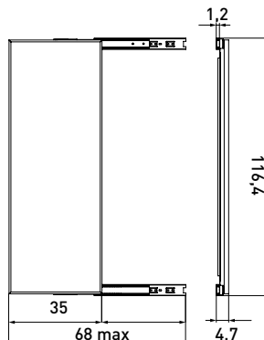
Espaciador para salvar bisagras incorporado
