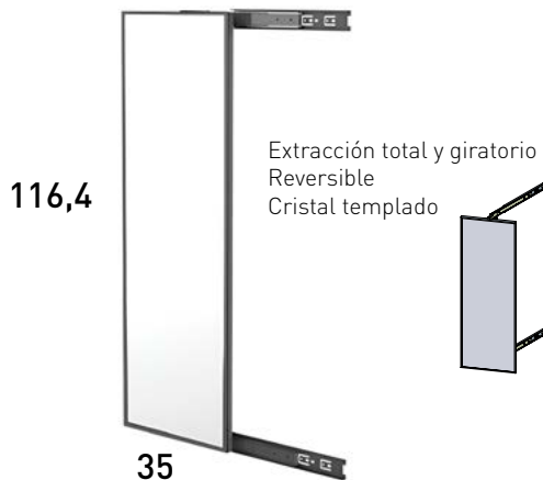
Espaciador para salvar bisagras incorporado
