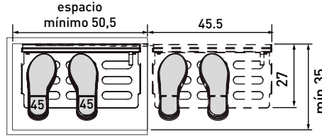
Espaciador para salvar bisagras incorporado
