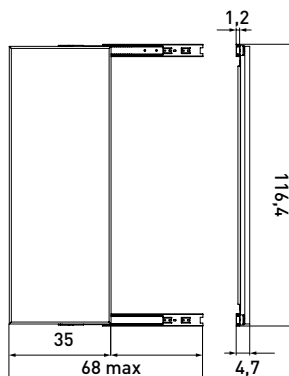
Espaciador para salvar bisagras incorporado
