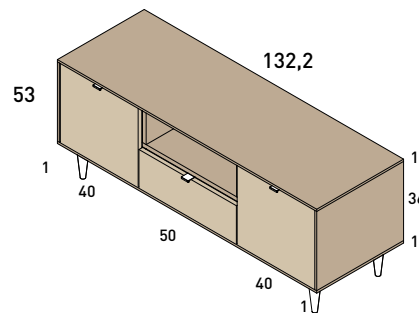
Tapa, base y forros de 1cm
