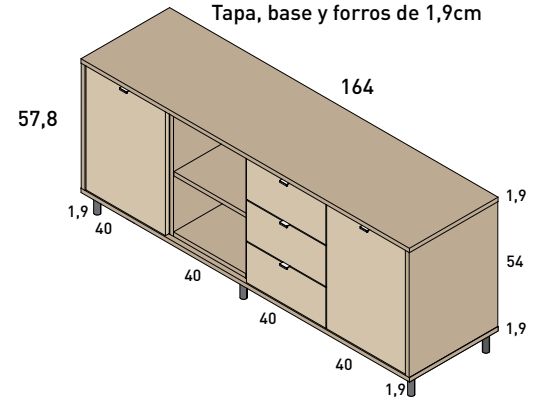
Tapa, base y forros de 1,9cm
