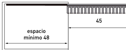
Espaciador para salvar bisagras incorporado
