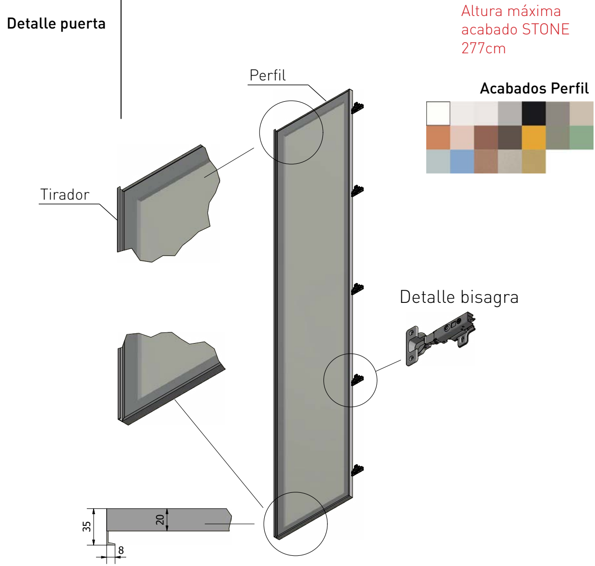
Ancho máximo de puerta 60 cm.
